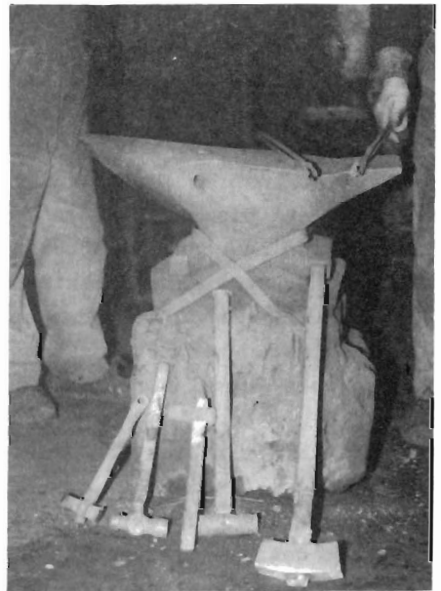
Zenbait erreminta ingudearen ondoan. Ezkerretik eskuinera, taieia, eskumailua, asentadera meharra, asentadera eta porra
